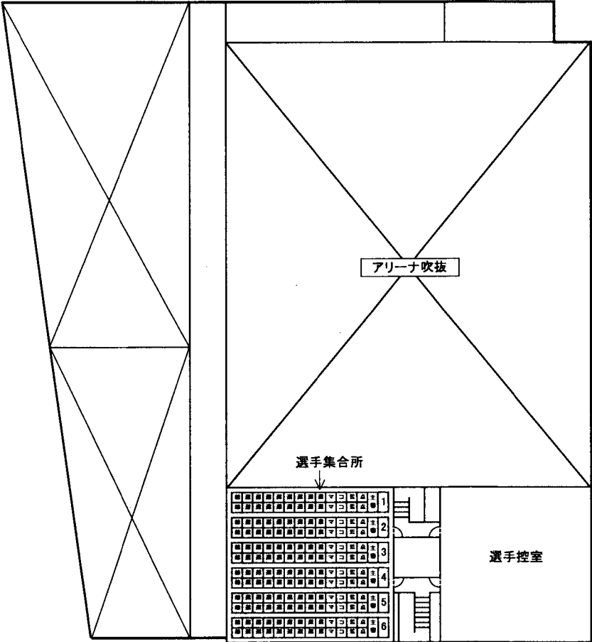
2F平面図
