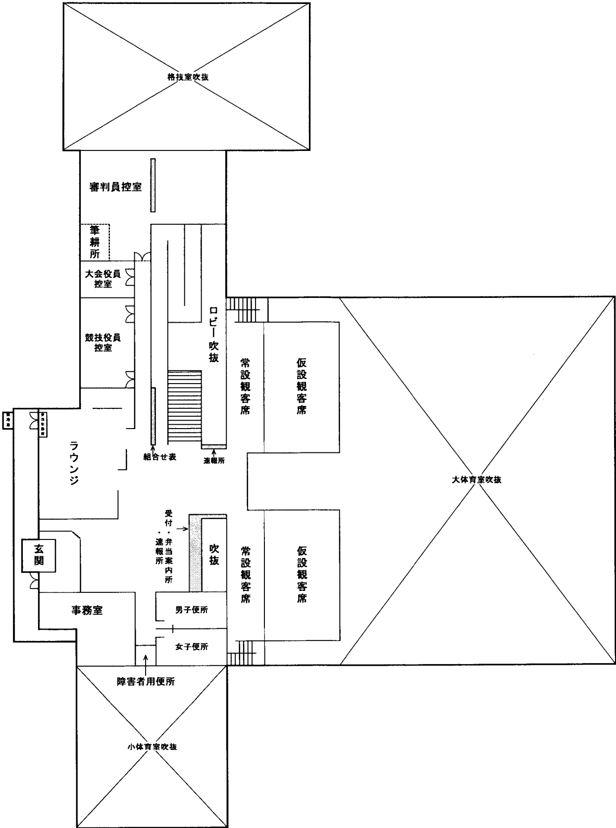
2F平面図
