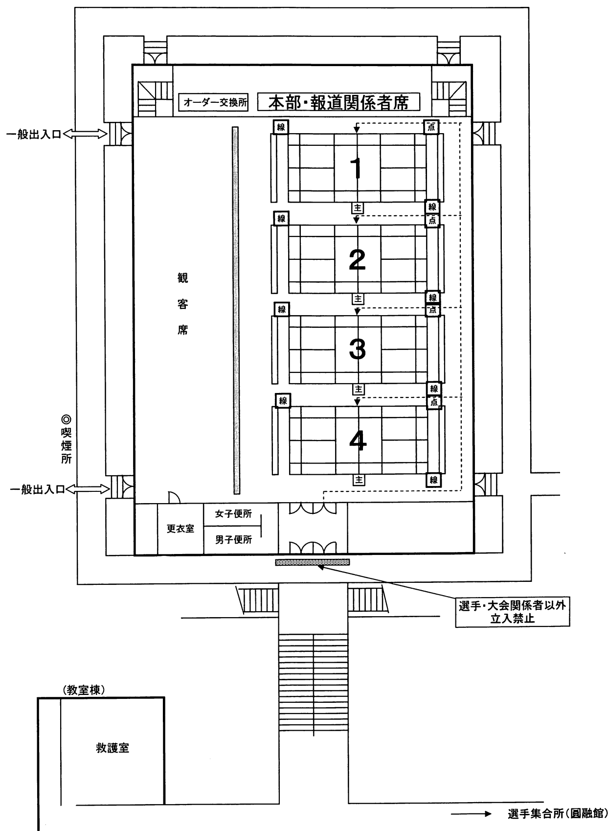
1F 平面図
