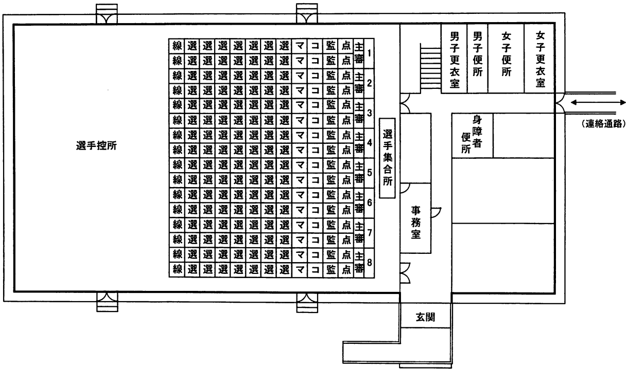
2F 平面図
