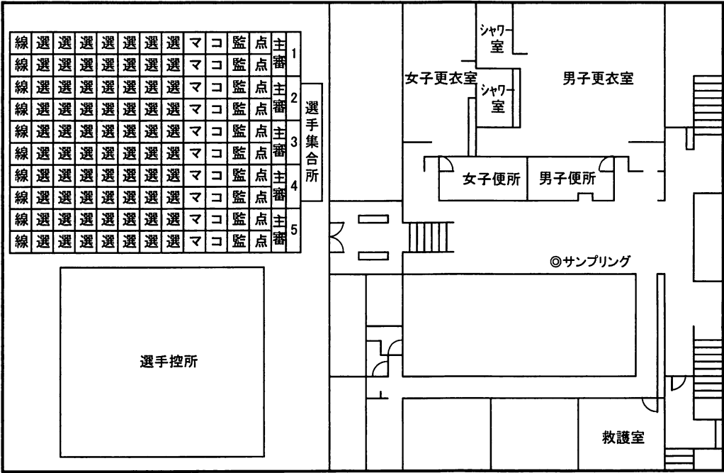
1F 平面図
