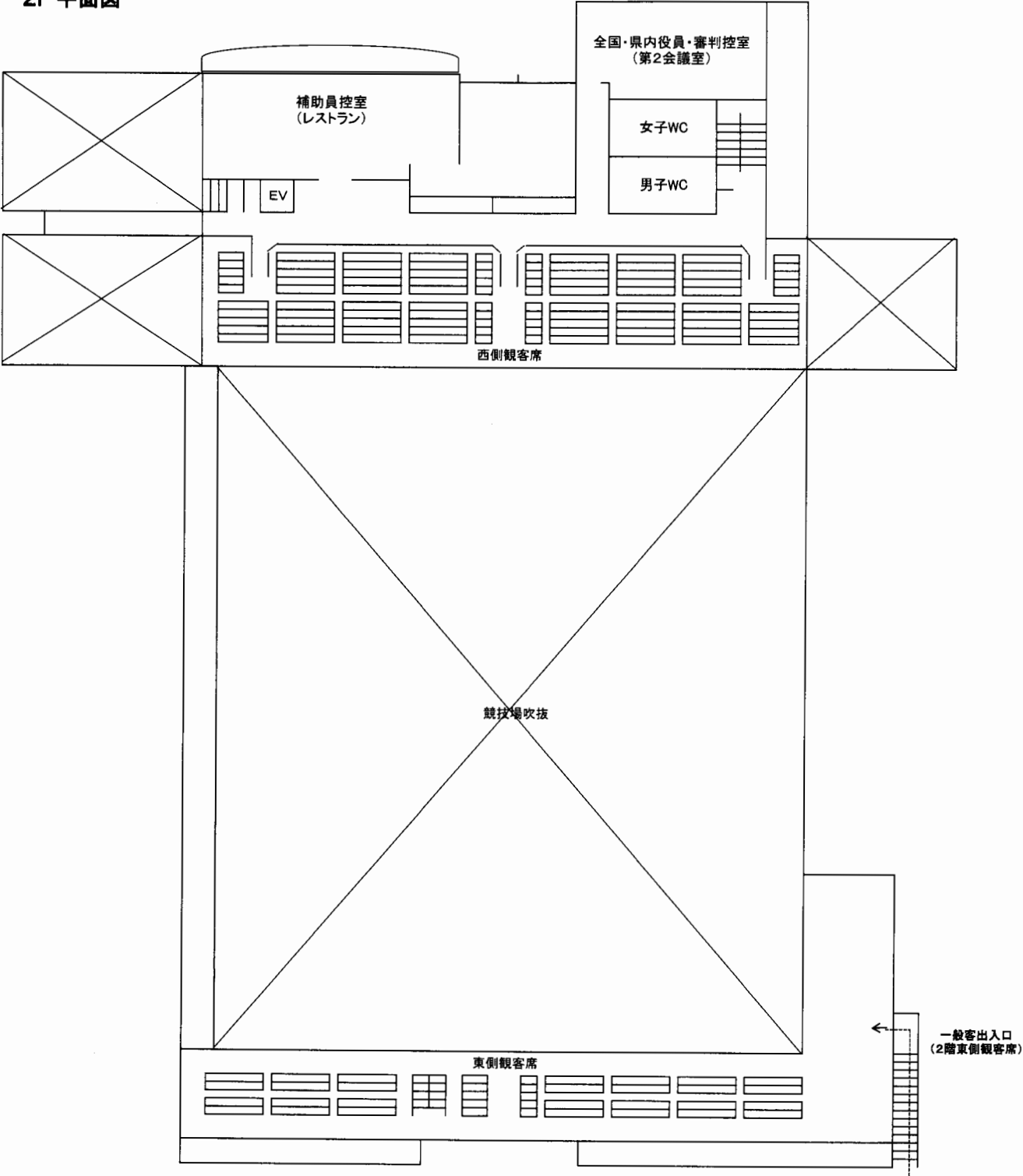
2F 平面図
