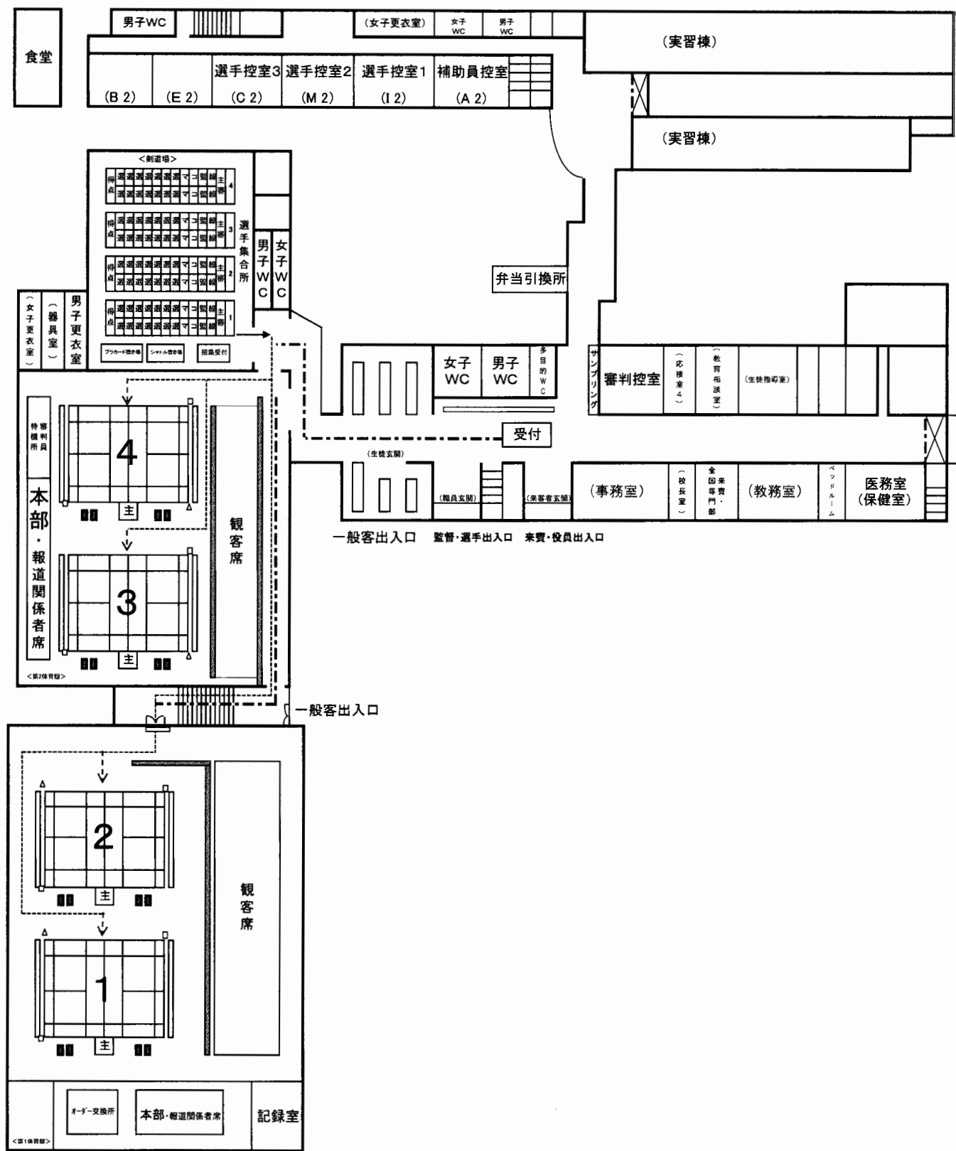
1F 平面図
