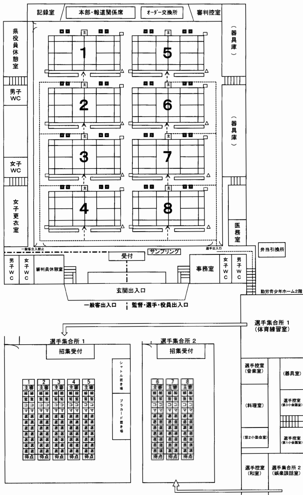
1F 平面图
