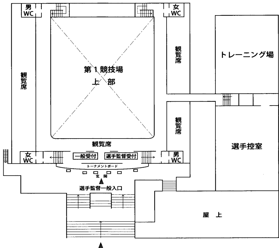
2 階平面図
